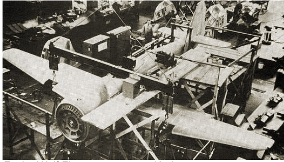
Focke-Wulf Flugzeugmontage 1942
